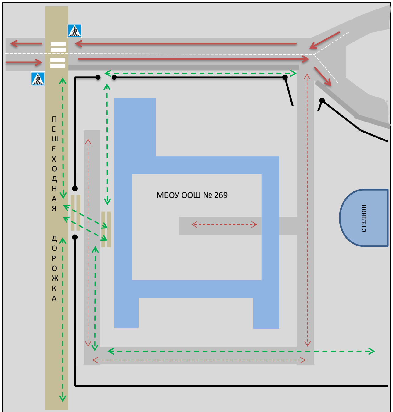
Схема организации дорожного движения в непосредственной близости от МБОУ ООШ № 269 с размещением соответствующих технических средств, маршруты движения детей.
